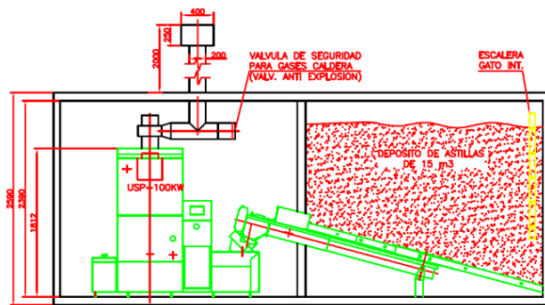
Diagrama de instalación
